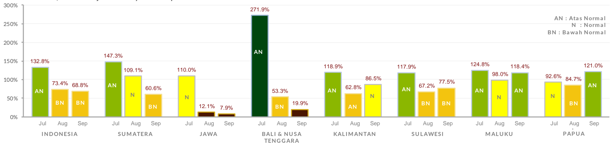
Analisis Sifat Curah Hujan Per Wilayah: Juli-September 2023
