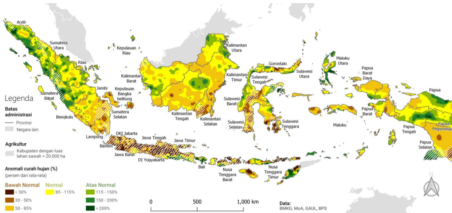
Analisis Sifat Curah Hujan Per Wilayah: Juli-September 2023
