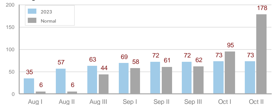
Jumlah zona musim yang mengalami Musim Hujan pada tahun 2023 dibandingkan dengan keadaan normal
